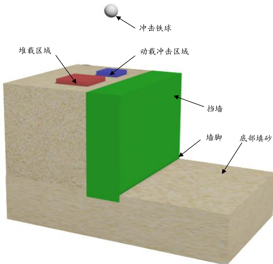
图 3 边坡加载示意图
